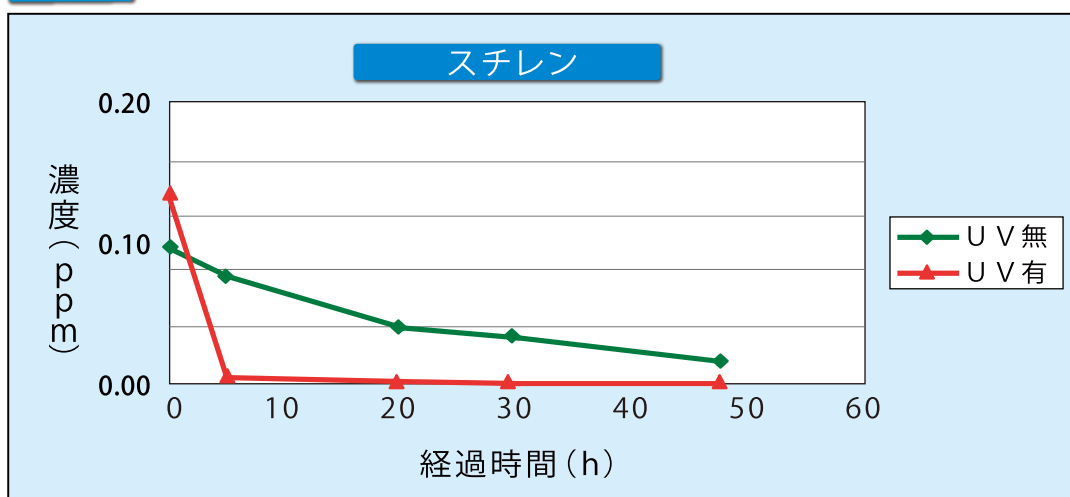
グラフ6 スチレンに対するトリニティー吸着・分解特性
