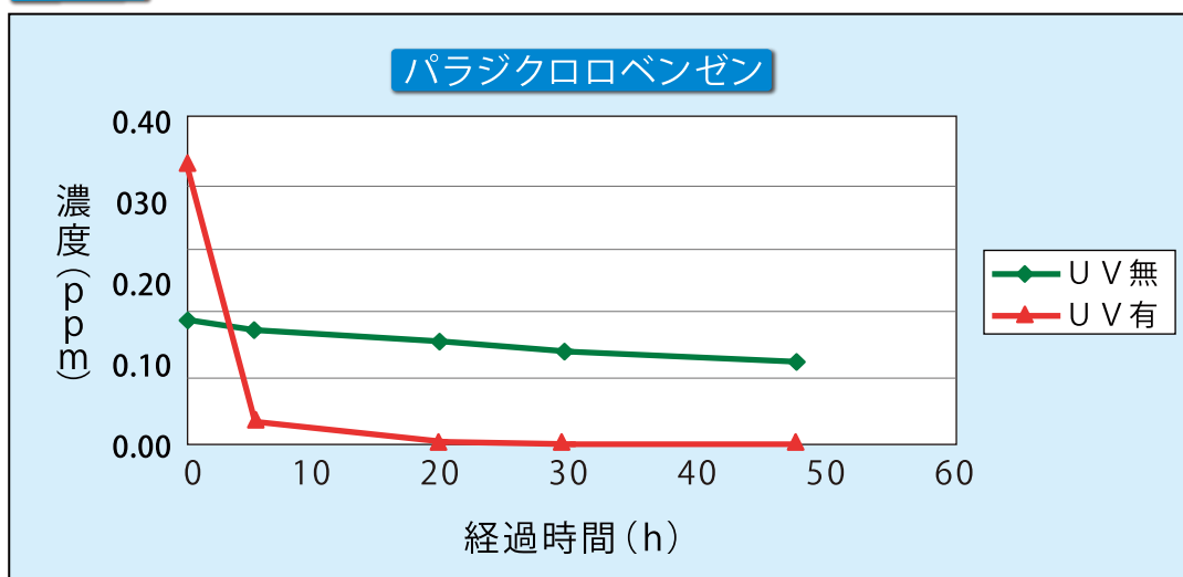
グラフ5 パラジクロロベンゼンに対するトリニティー吸着・分解特性
